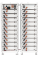
BOS-A
